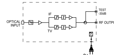
Diagrama de Bloques Block Diagram Schéma Synoptique
